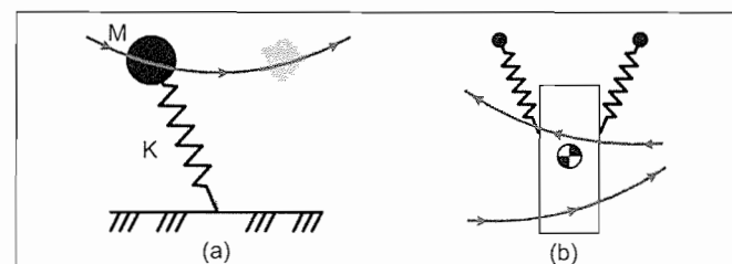
圖2 運動模型：(a)生物水平運動時使用之簡化模型：彈性倒擺模型 [52] ；(b)生物動態爬牆時可使用之簡化模型 [60] 。
