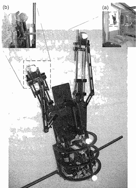
圖3 二足動態爬牆機器人DynaClimber：(a)實驗環境設定；(b)爪部放大圖。
