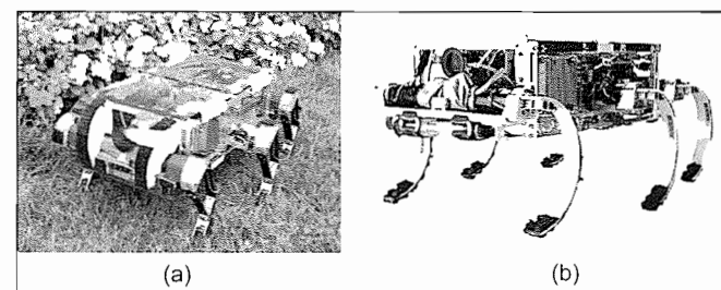
圖1 六足機器人RHex：(a)配備1D被動自由度之四連桿撓性腳；(b)配備2D被動自由度之半圓撓性腳。
